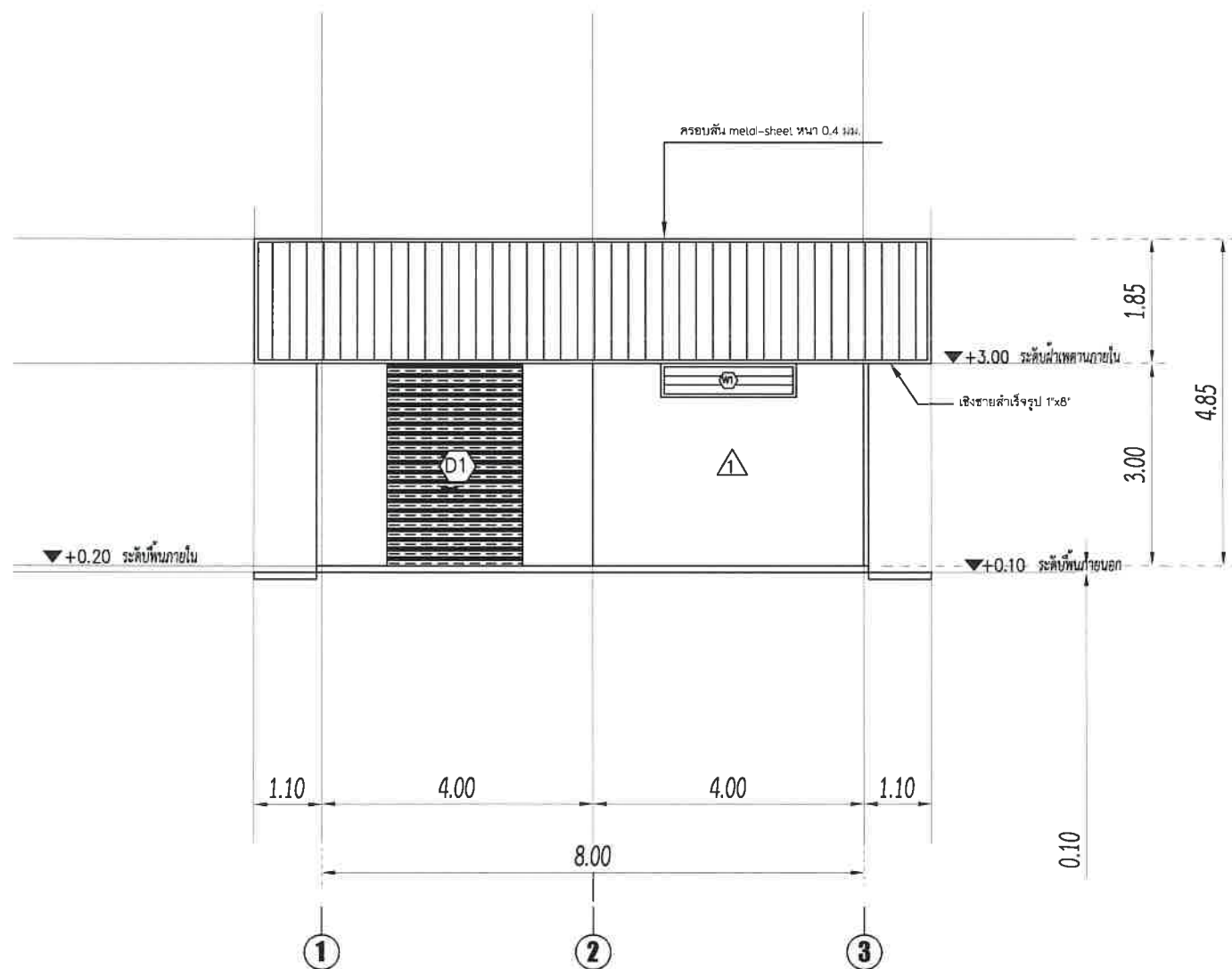
รูปด้าน 1 SCALE 1 : 100
