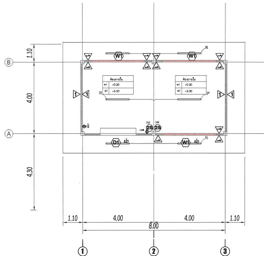
ผังไฟฟ้าแสงสว่าง SCALE 1 : 100
