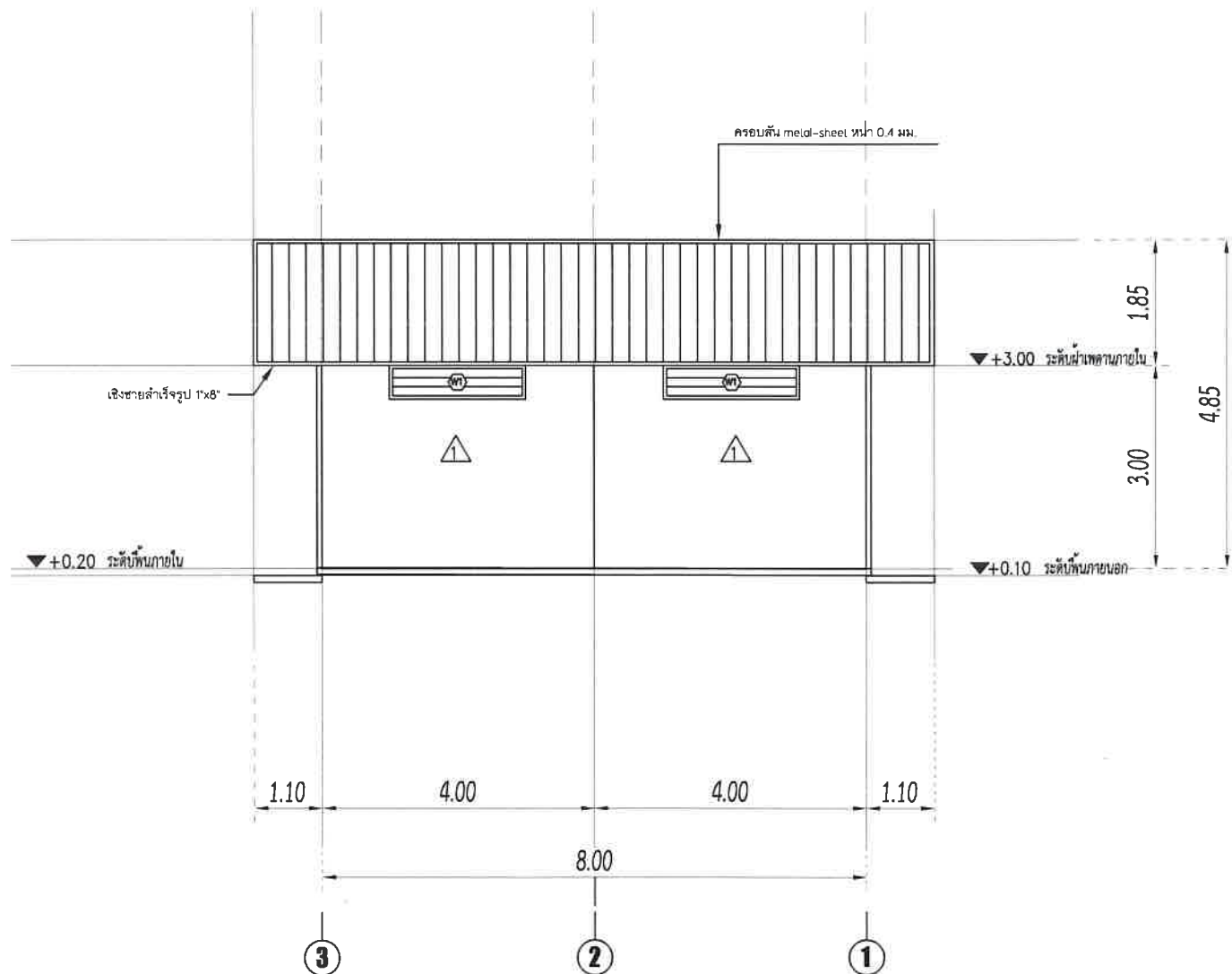
รูปด้าน 4 SCALE 1 : 100
