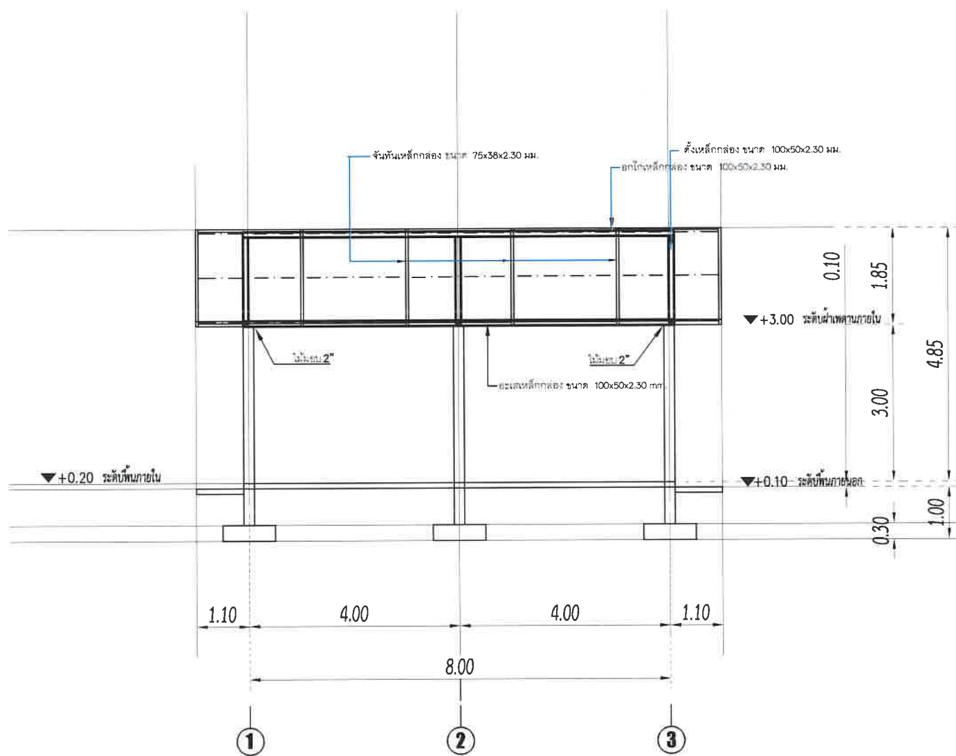
รูปตัด A-A SCALE 1 : 100
